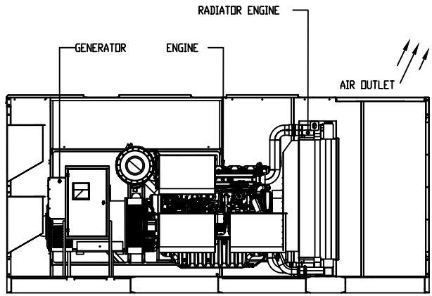
SECCION B-B ESCALA 1 : 30
